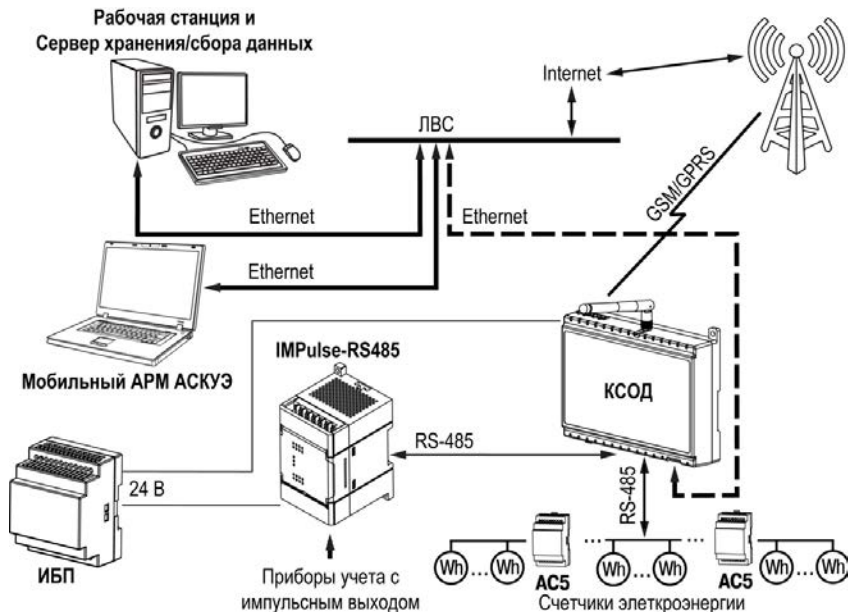
Рисунок 6.2 – Пример структуры соединений при использовании KCOD в системе управления
